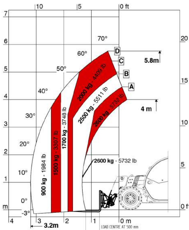
DIAGRAMA DE CARGA
