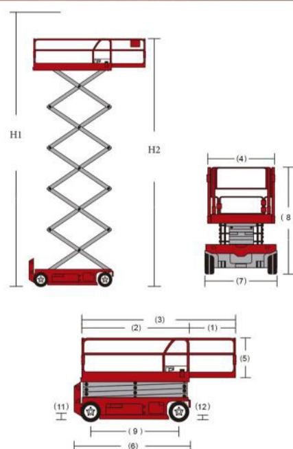
Diagrama dimensiones
